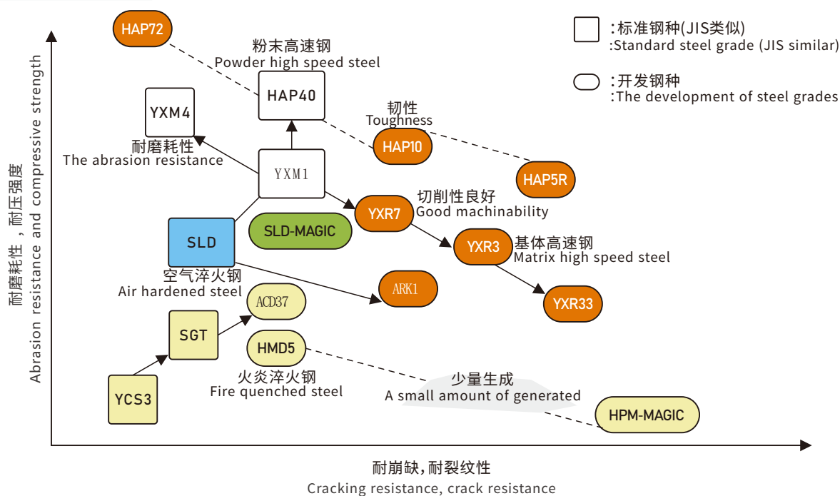
各种钢种的特殊关系图
